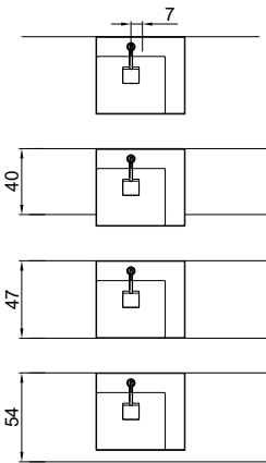
schema d' installazione lavabi e rubinetteria / sinks and taps installation layout
